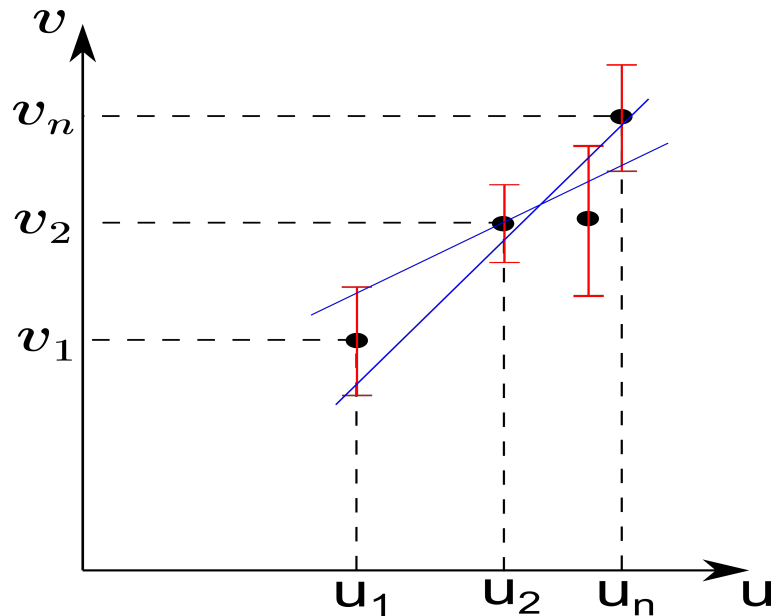
Рис. 9.5: Построение прямой через точки, заданные с ошибкой
