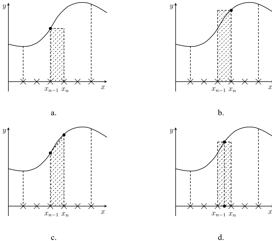
Рис. 3.2: геометрическая интерпретация формул: а) левых прямоугольников, б) правых прямоугольников, в) трапеций, д) средних прямоугольников.
