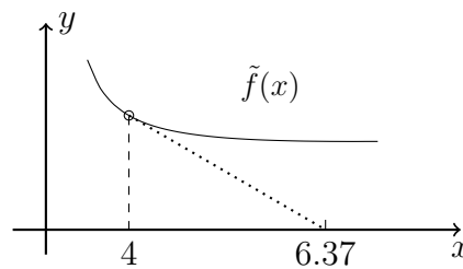
Рис. 1.5: Поиск последнего корня.
