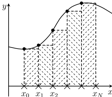
Рис. 3.5: формула левых прямоугольников с узлами, упорядоченными слева направо.
