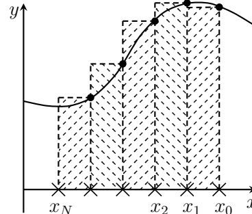
Рис. 3.6: формула левых прямоугольников с узлами, упорядоченными справа налево.
