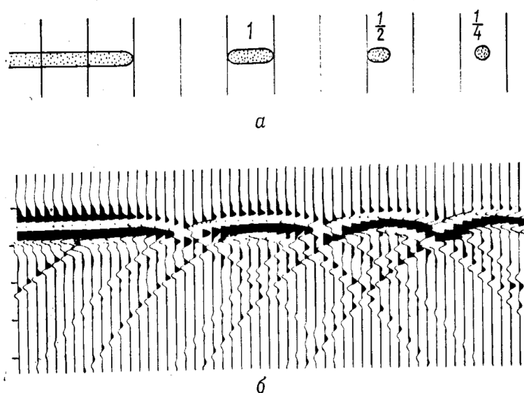
Рис. 6.10. Отражение от тонкого пласта ограниченной протяженности. Протяженность
