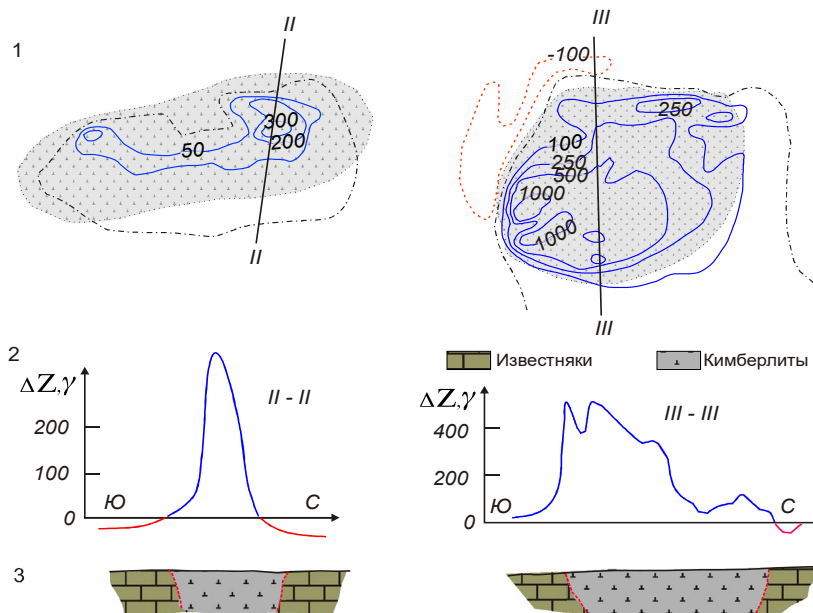
Рис. 4.10. Применение магниторазведки при поисках кимберлитов. Примеры магнитных аномалий трубчатого типа. 1 – планы изодинам, 2 – графики \Delta Z, \gamma , 3 – геологические разрезы
