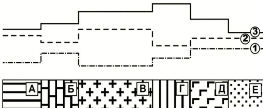
Рис. 1.3. Физико-геологическая ситуация 3
