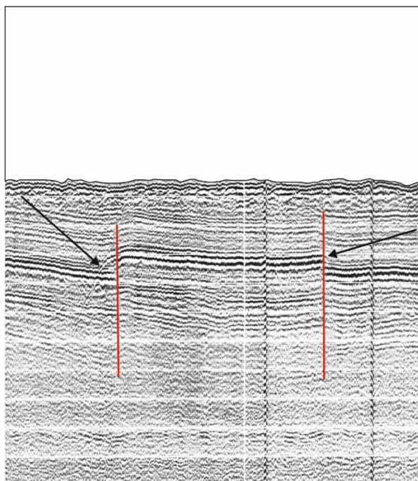
Рис. 7.15. Образование дифрагированных волн в зонах разрывных нарушений
