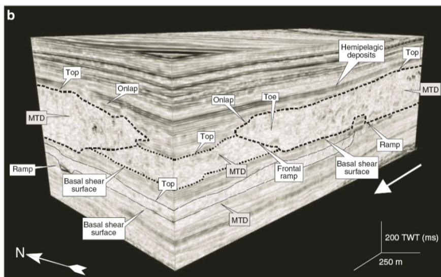
Рис. 7.11. 3D визуализация Mass Transport Deposites (MTD)
