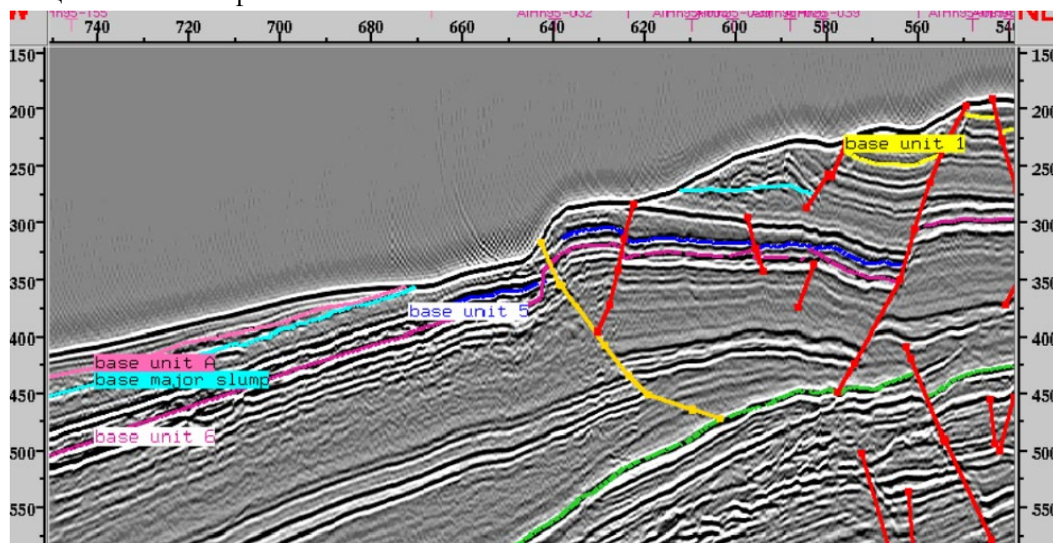
Рис. 7.9. Сейсмический профиль через оползень с вращением
