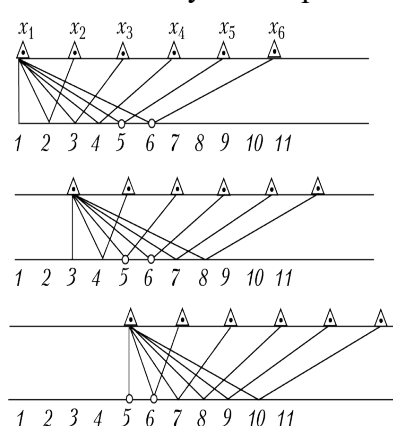
Рис. 6.15. Схема полевых наблюдений МОГТ, обеспечивающая перекрытие по ОГТ
