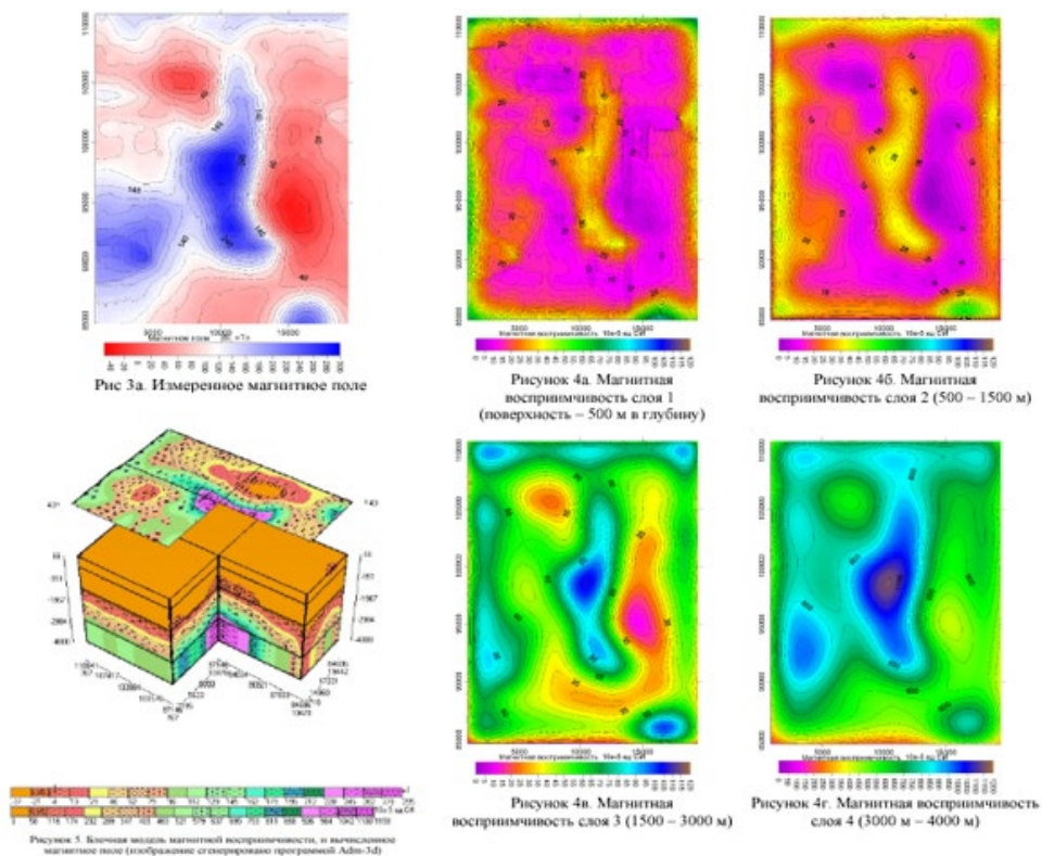
Рис. 4.9. Высокоточная магниторазведка при изучении нефтесперспективных участков. Муравьев Л.А. Институт геофизики УрО РАН (450 кв.км. 30 дней)
