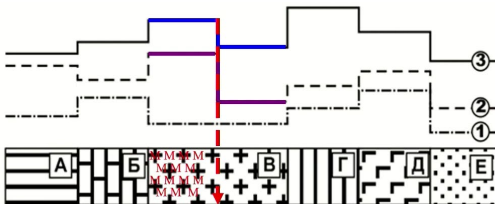
Рис. 1.4. Физико-геологическая ситуация 4
