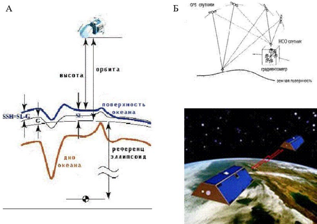
Рис. 2.6. А – спутниковая альтиметрия, Б – спутниковая гравиметрия
