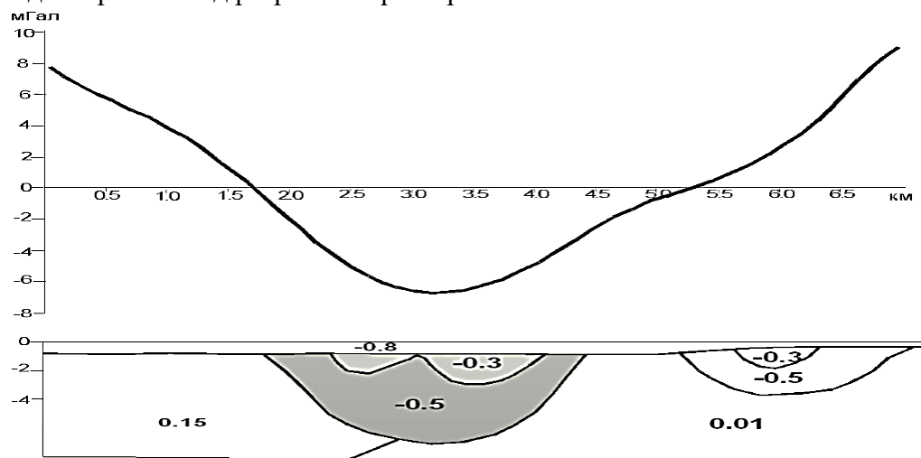
Рис. 1.5. Плотностной разрез
