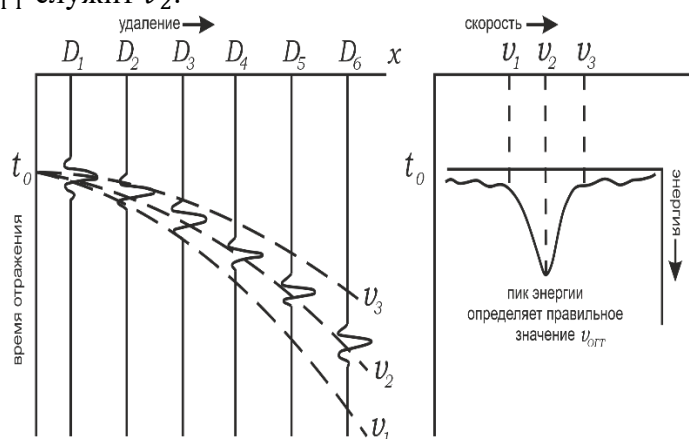
Рис. 6.16. Кинематический сдвиг
