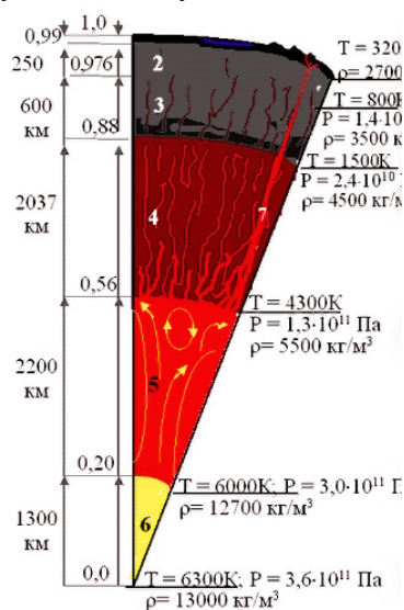
Рис. 3.4. Строение Земли
