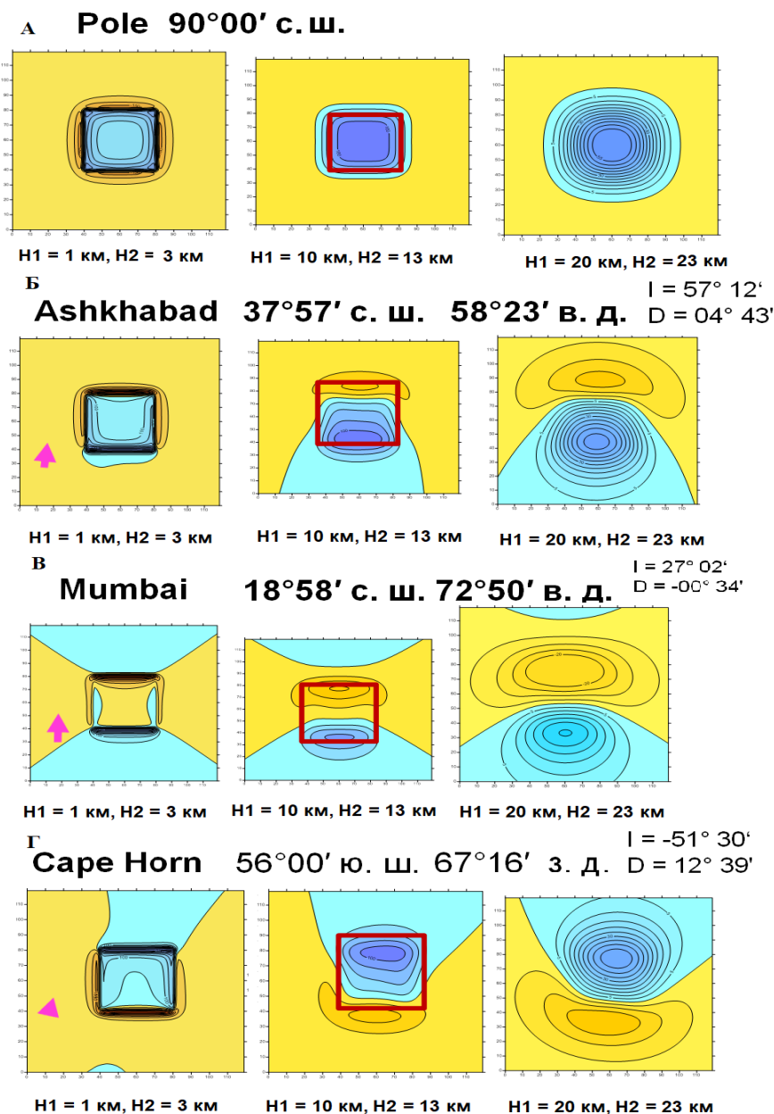
Рис. 4.6. Структура магнитной аномалии
