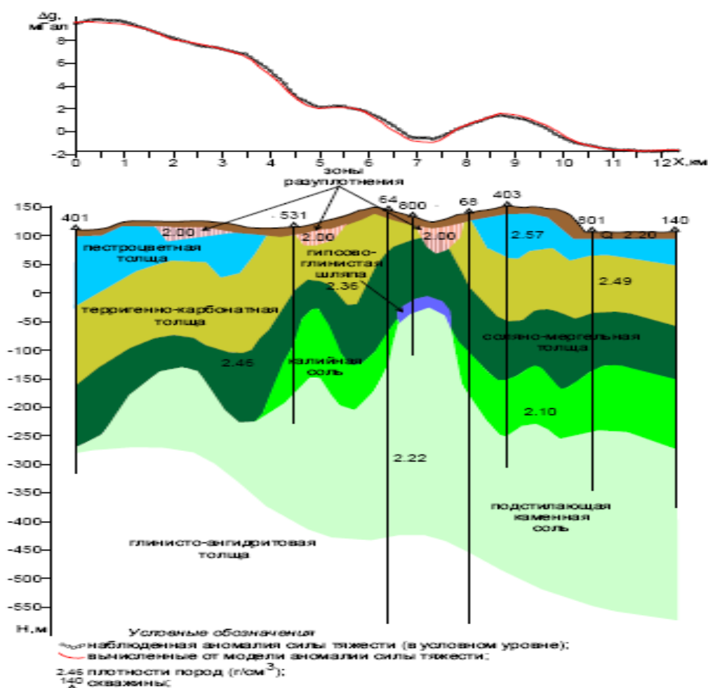
Рис. 3.8. Результат интерпретации гравитационного поля Шершевского соляного месторождения (По данным Бычкова С.Г.). Горный институт УрО РАН, Пермь 2005
