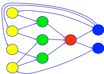
Рис. 10: Периодическая цепь с периодом 4: из состояний каждого цвета можно попасть только в состояния следующего цвета
